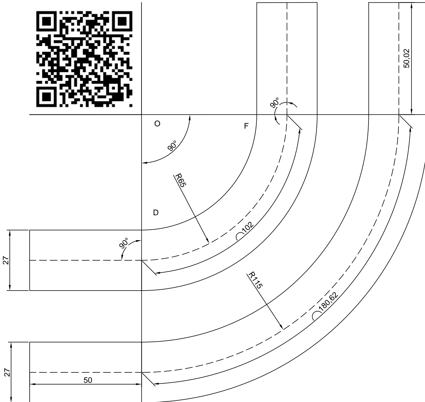
COUDE À EPOUSEMENT ( OU COUDE CONCENTRIQUE) RC (RAYON CINTRAGE) 115 mm TUBE ACIER 3/4" 20X27
